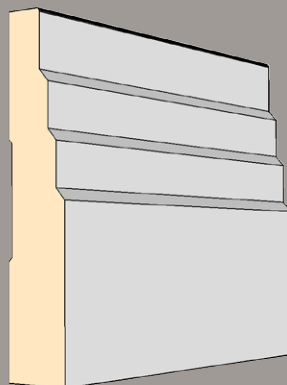
Talía Skirting EDM 2005 140x18
